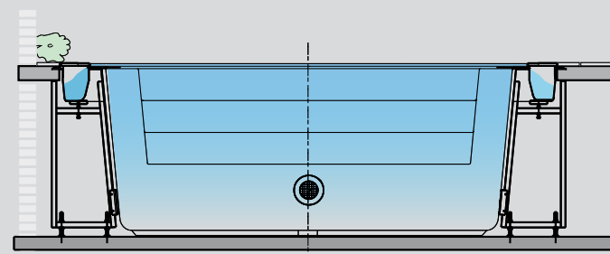
Einbau freitragend mit Überlaufrinne: Wandverstreben aus Stahl.
