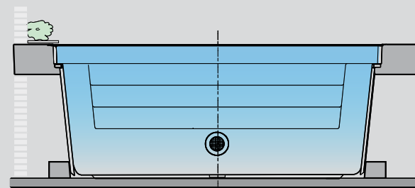
Einbau als freitragende Variante: Wandverstreben anlaminiert.
